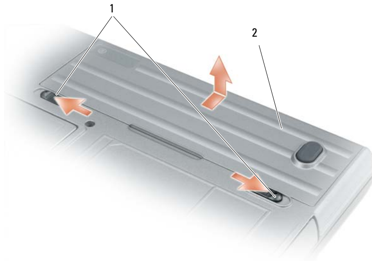
1 電池凹槽釋放門鎖 2 電池
